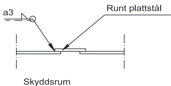
Figur T04-301b. Sektion genom dörrblad efter åtgärd.
